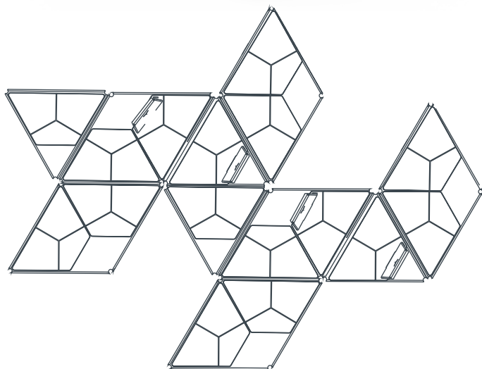
YPSILON 5 ÖSSZEÁLLÍTÁS
